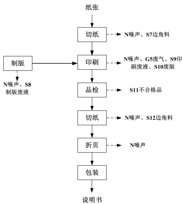
图 2-3 说明书生产工艺流程及产污环节图
