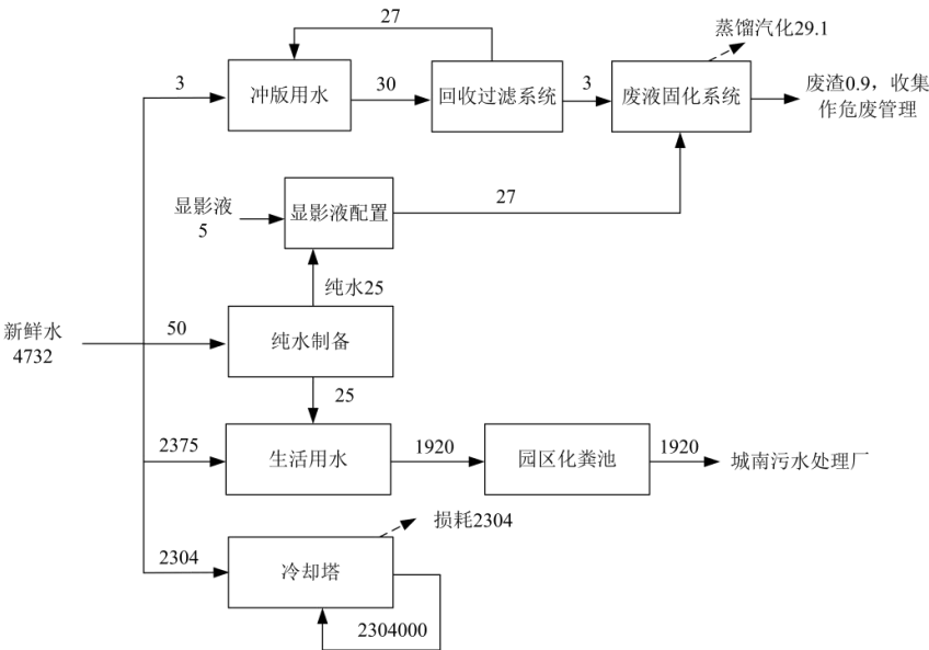
图 2-1 本项目水平衡图 (t/a)
