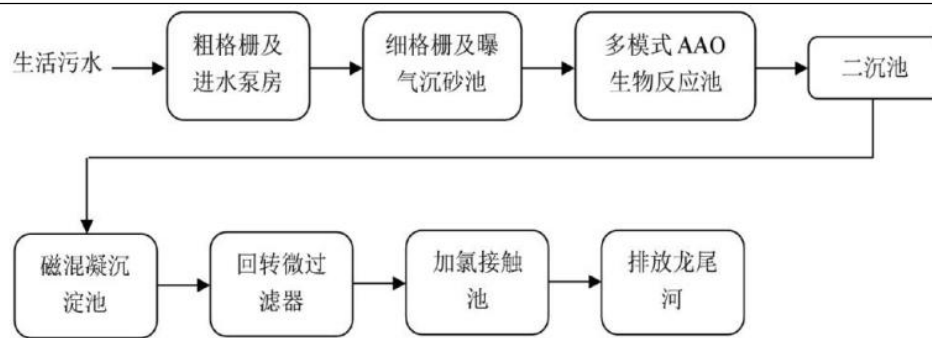
图 4-2 城南污水处理厂处理工艺流程图（二期）
