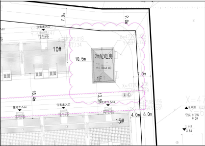
2# 配电房调整后
