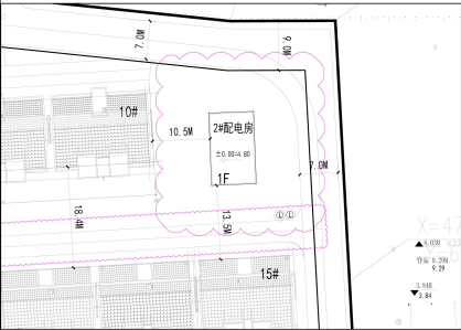
2# 配电房调整前
