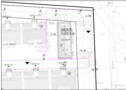
3# 配电房调整后
