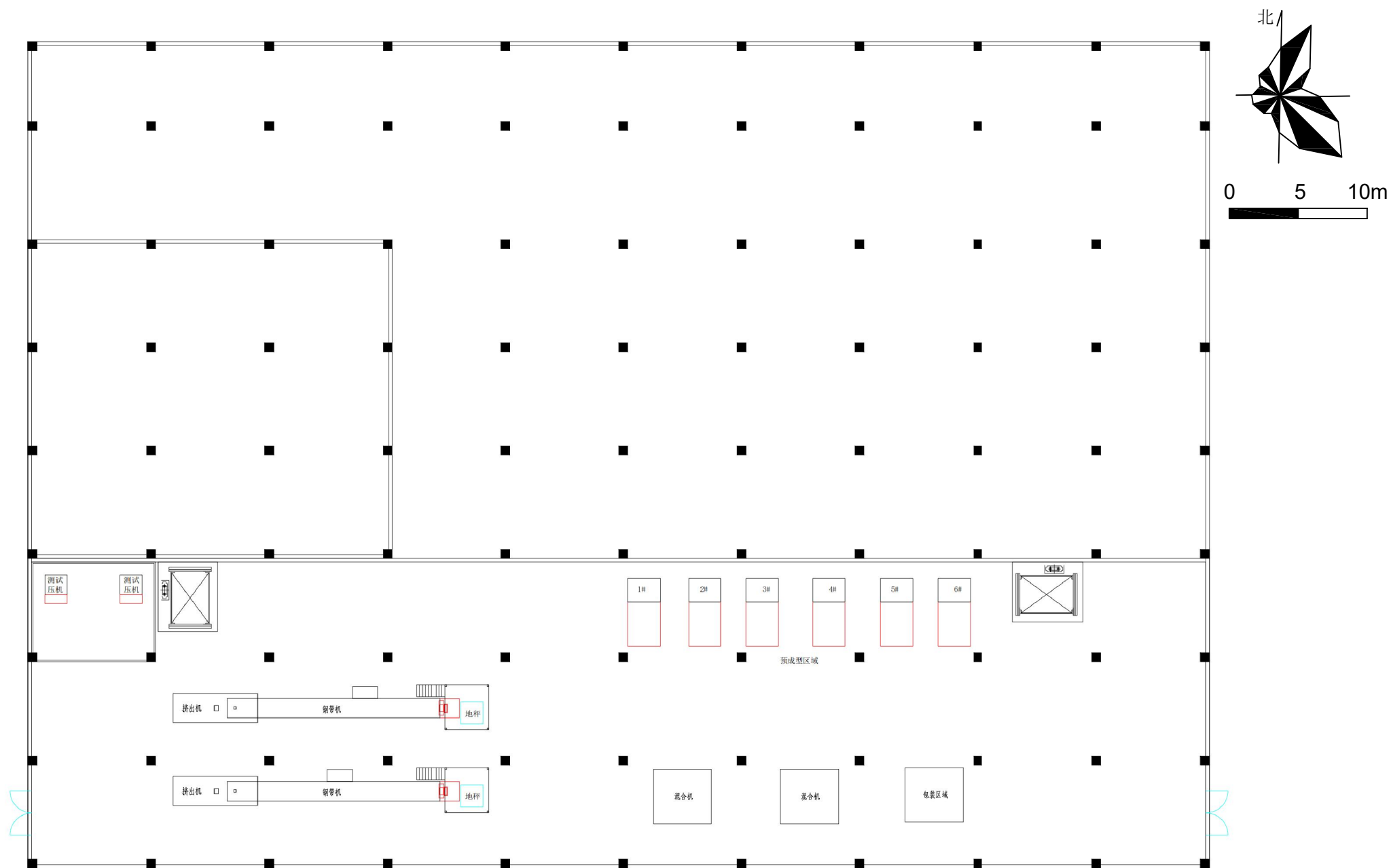
附图3-2 建设项目平面布置图（车间1楼）
