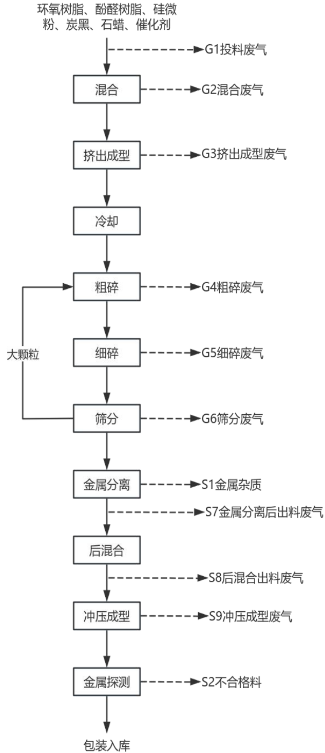
图 2-4 生产工艺流程图
