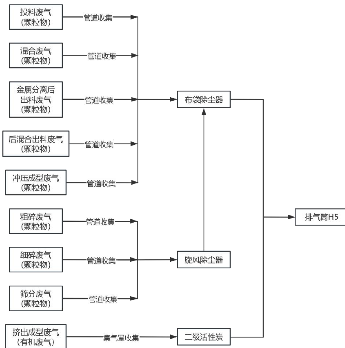
图 7.1-1 项目废气处理措施走向图
