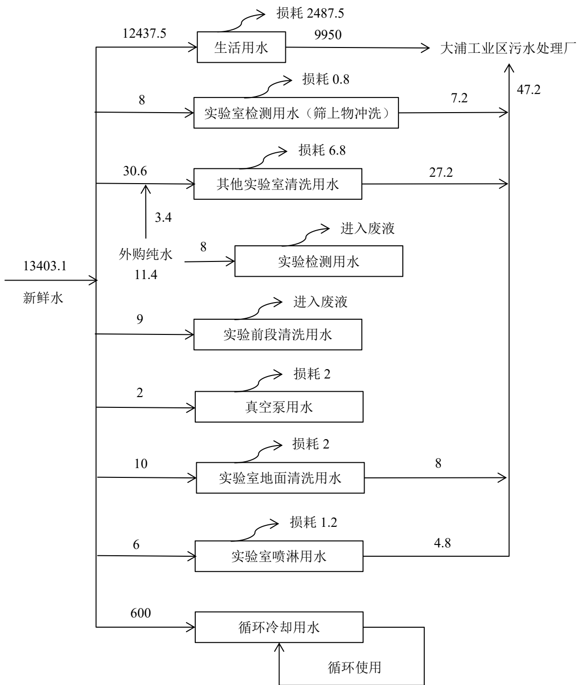
图 2-3 本项目建成后二部厂区水平衡图（单位： \text{m}^3/\text{a} ）
