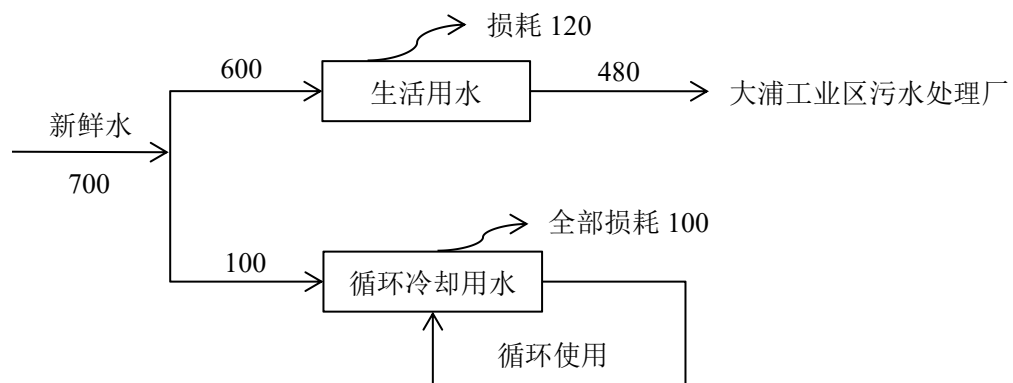
图 2-2 本项目水平衡图（单位： \text{m}^3/\text{a} ）
