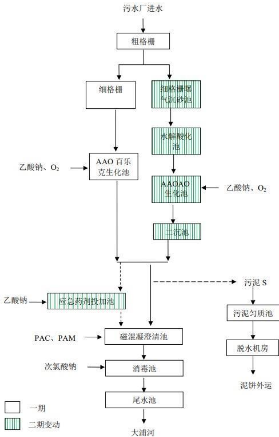
图 4-1 恒隆污水处理厂污水处理工艺流程图
