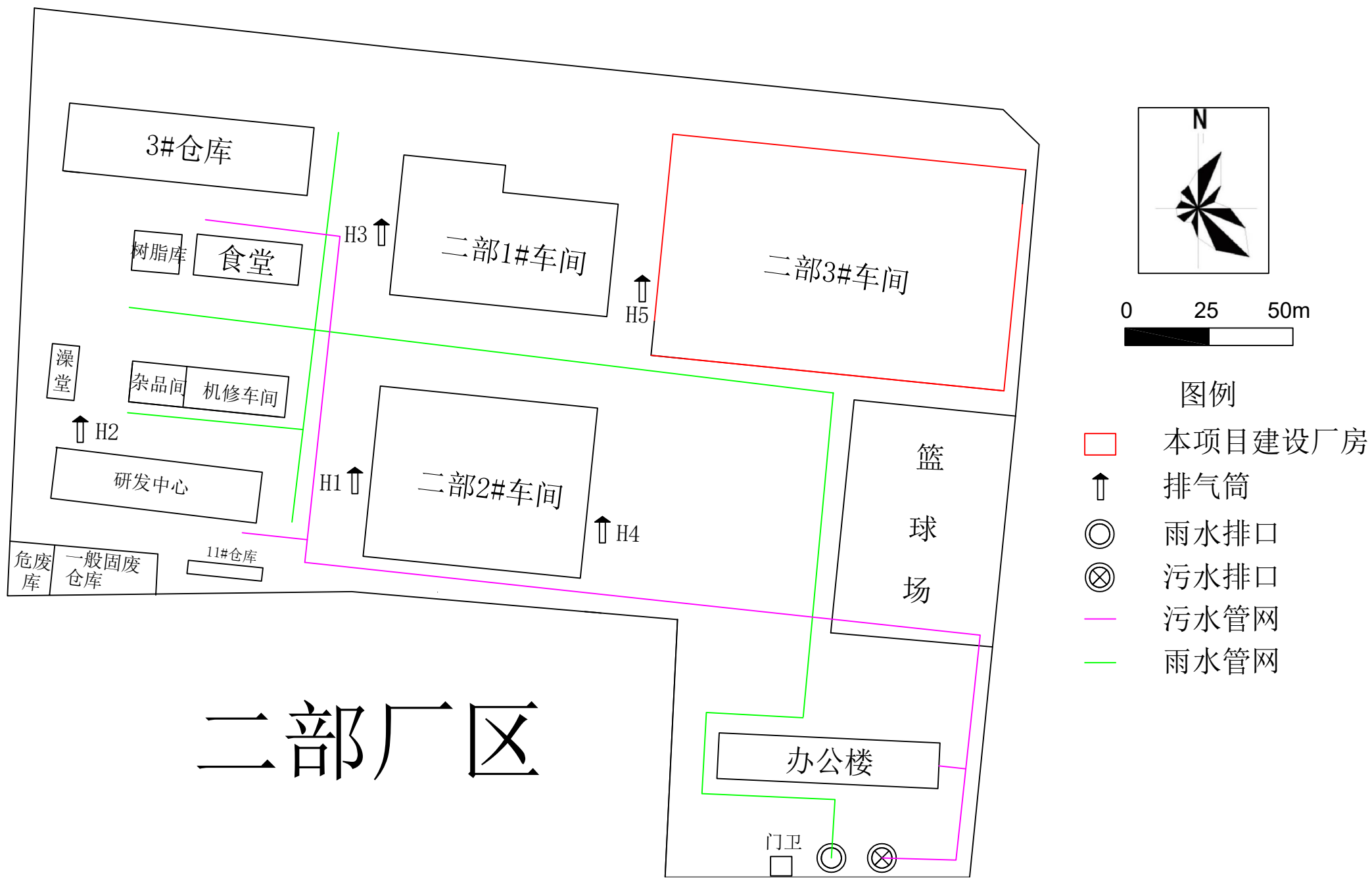
附图3-1 二部厂区平面布置图
