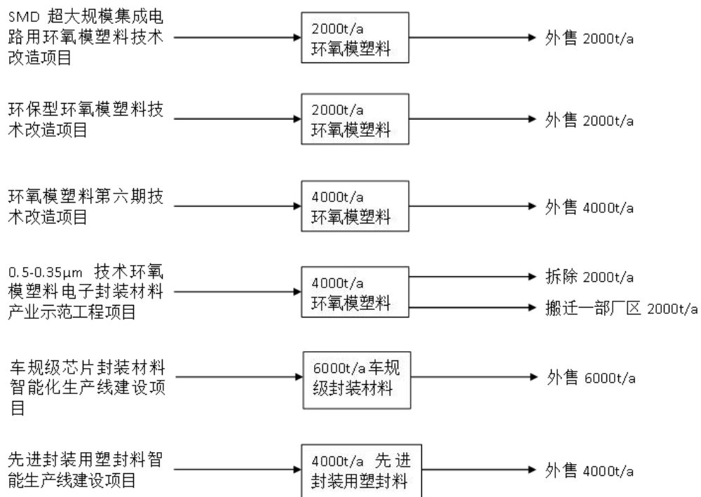
图 2-1 本项目建成后二部厂区产品上下游关系图
