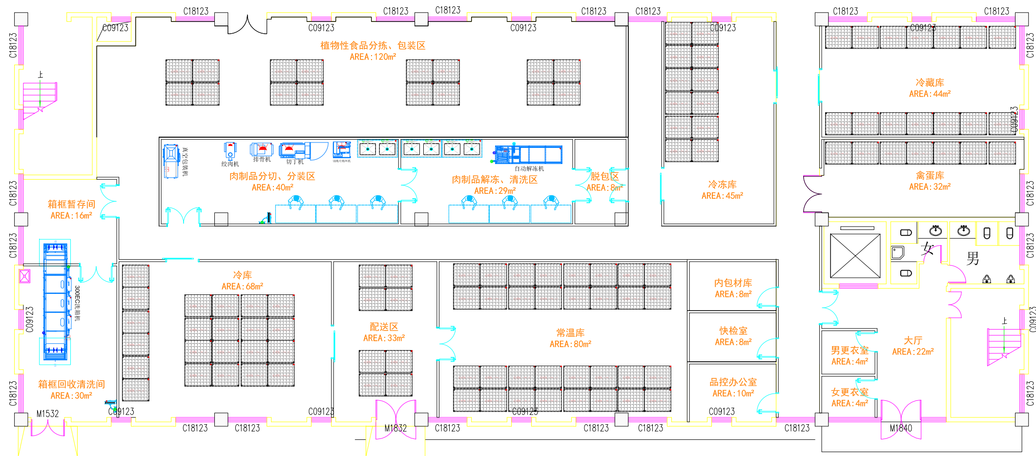
附图3-2 3号车间一层平面 (1:200)
