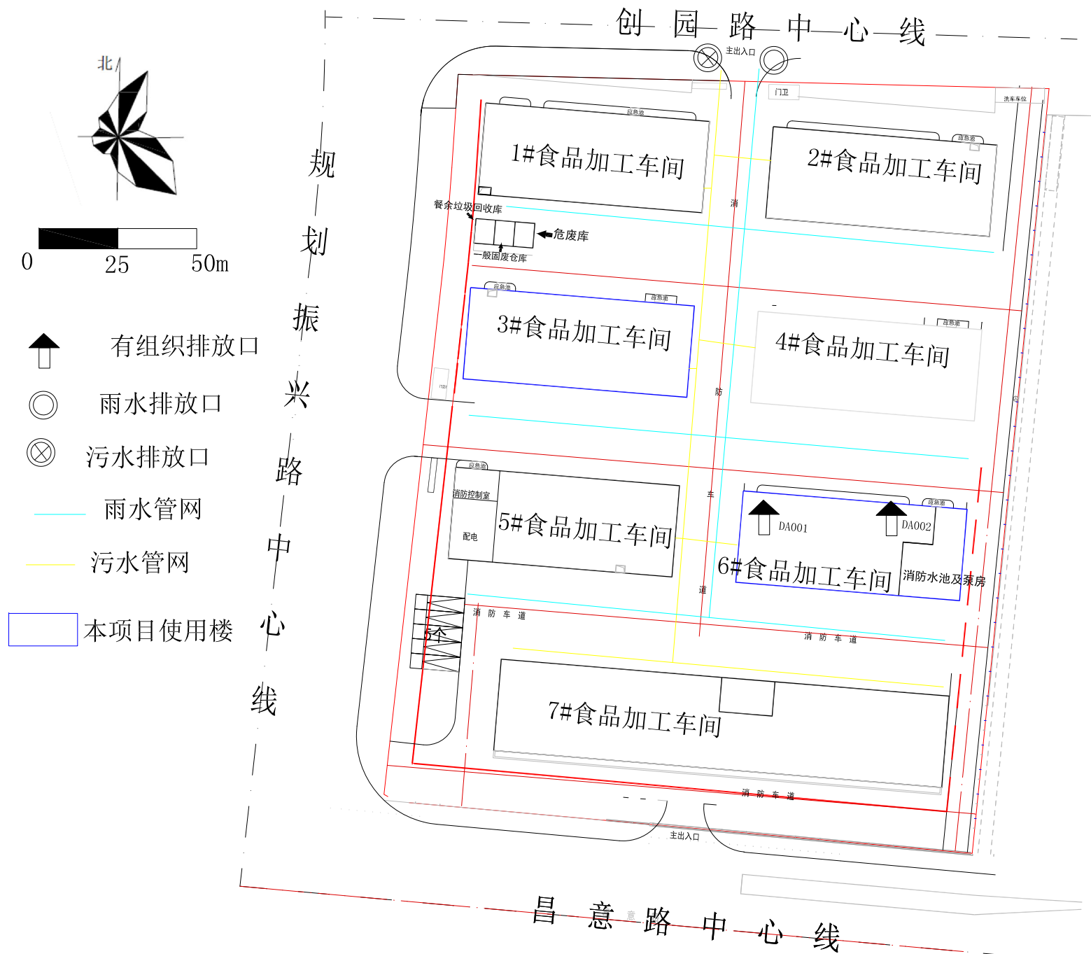
附图3-1 厂区总平面布置图
