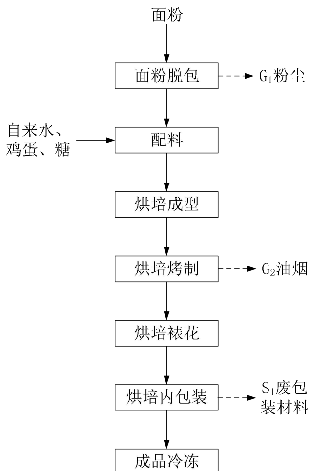
图 2-4 烘焙类工艺流程及产污节点示意图
